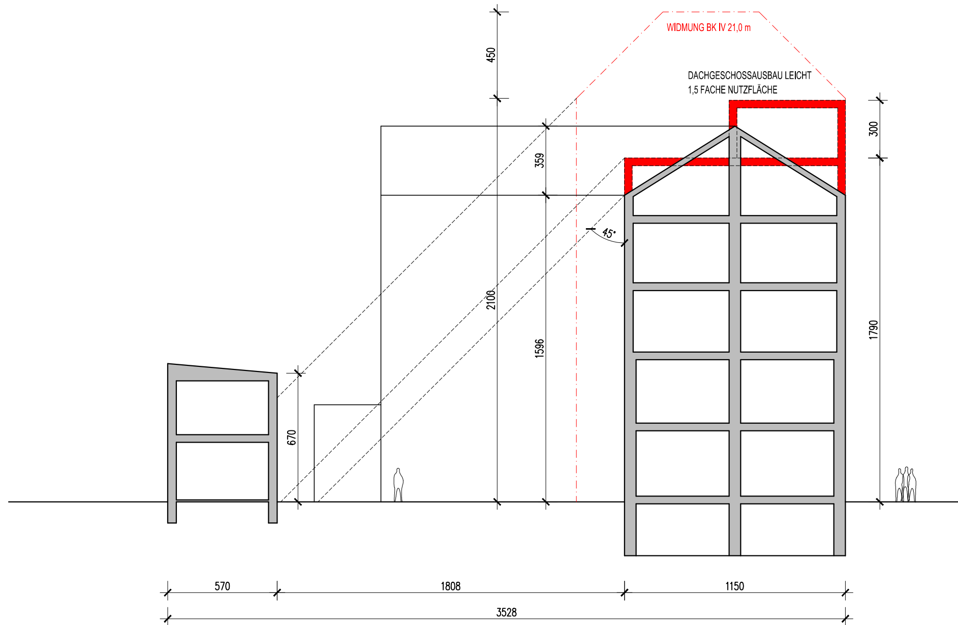
SCNITT A-A
